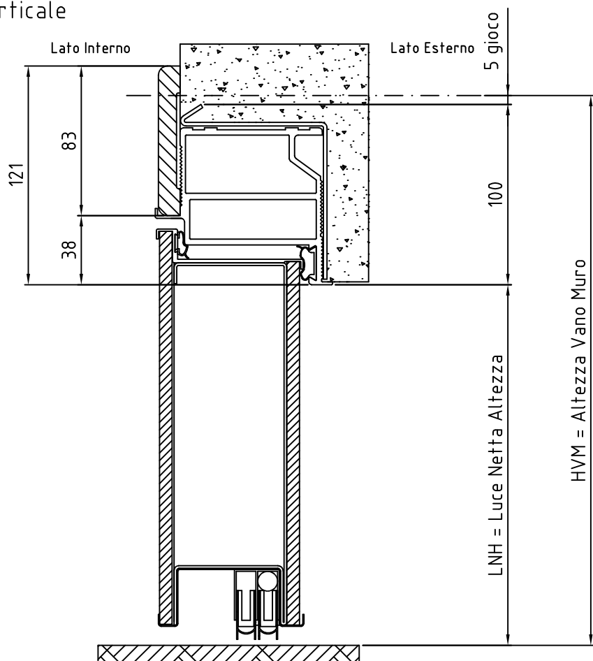
Sez. Verticale
