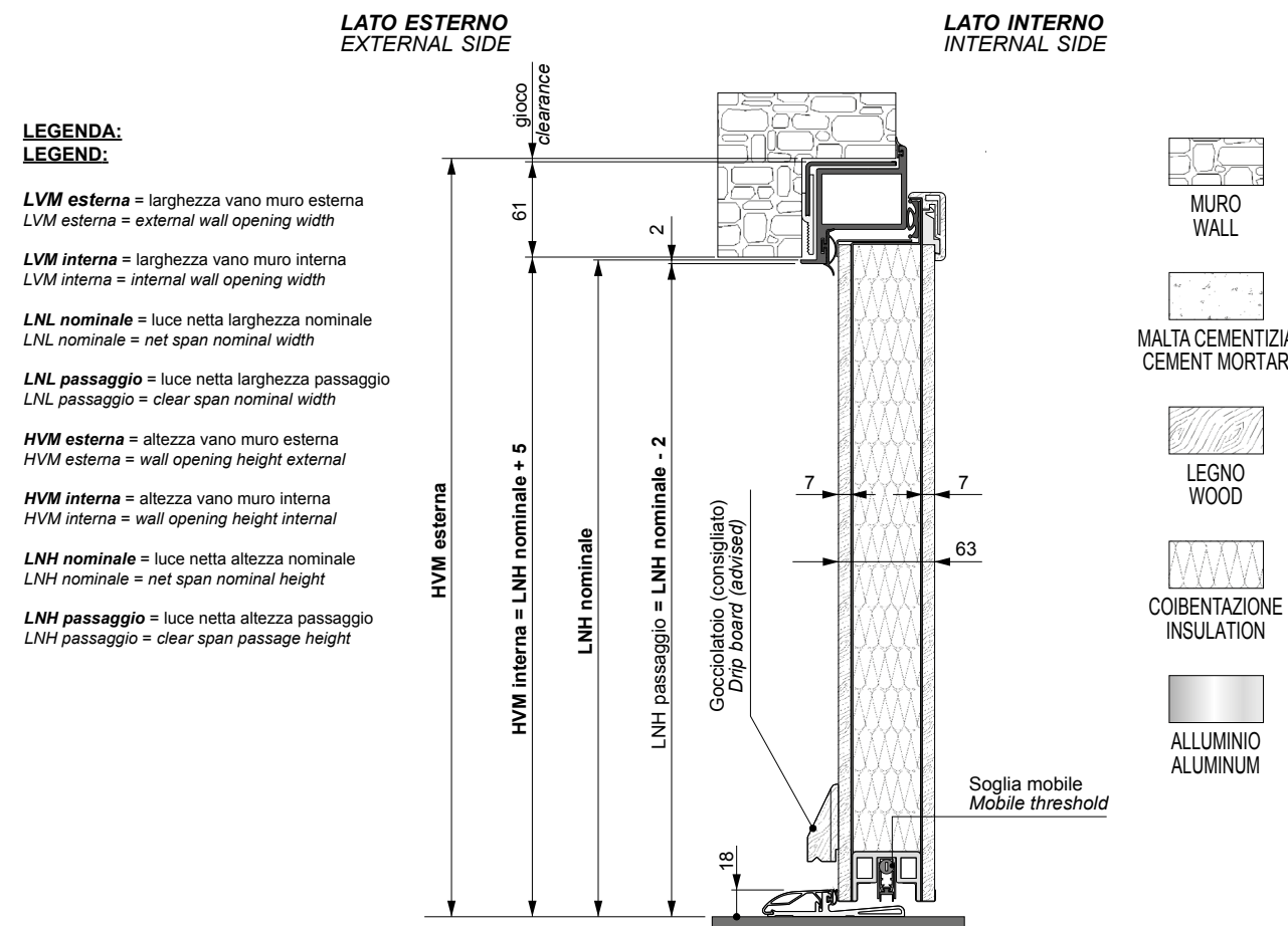
SEZIONE LONGITUDINALE - LONGITUDINAL SECTION -
