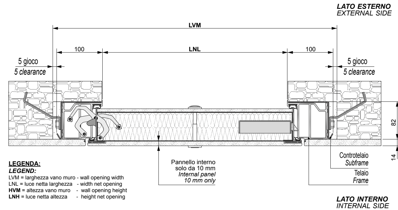
SEZIONE TRASVERSALE - CROSS SECTION -
